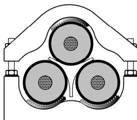
Med elastiskt inlägg och avståndskil för högspända oljekablar och vid vertikalt montage
